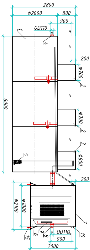
Разрез 1-1
